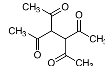
Bis(acetylacetone) CAS RN: 5027-32-7
