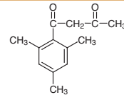
1-(2-Mesitylene)- 1,3-butanedione CAS RN: 6450-57-3
