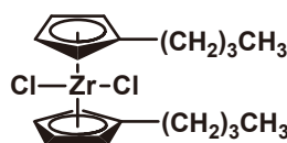
1,1'-Dibutylzirconocene Dichloride
