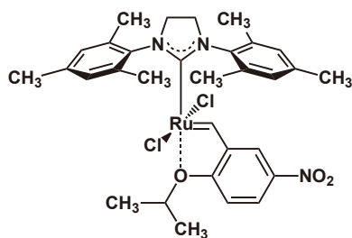
nitro-Grela 100mg / 500mg [N1060]
