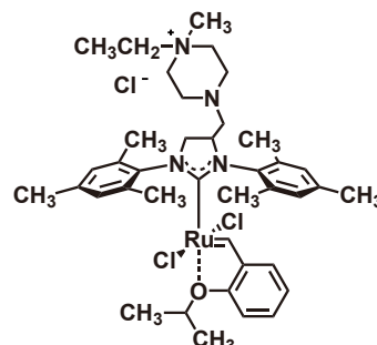
AquaMet 100mg / 500mg [A3009]
