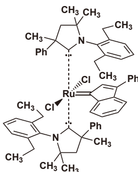
UltraCat 100mg [U0141]
