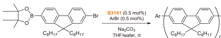
Bis(tri-tert-butylphosphine)palladium(0)
