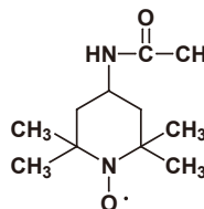
4-Acetamido-TEMPO Free Radical
