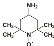
4-Amino-TEMPO Free Radical
