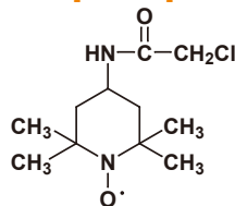
4-(2-Chloroacetamido)-TEMPO Free Radical
