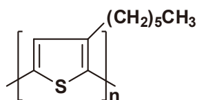
P3HT
