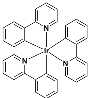
Ir(ppy) 3 200mg / 1g [T3716]
