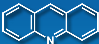
Acridine
