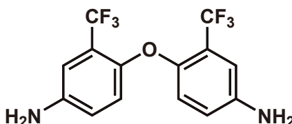
6-FODA
