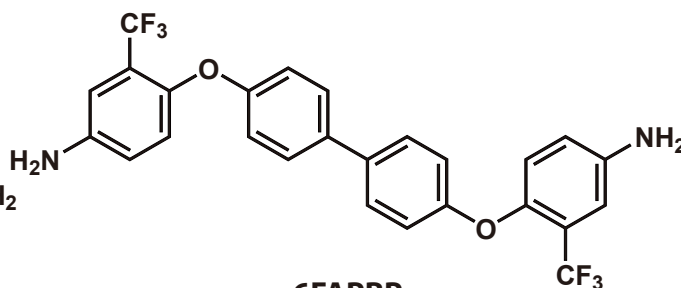
6FAPBP
