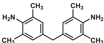
MBDA
