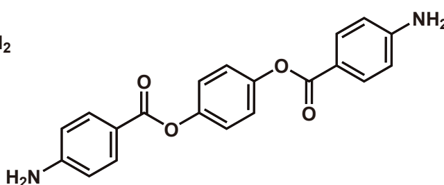
ABHQ
