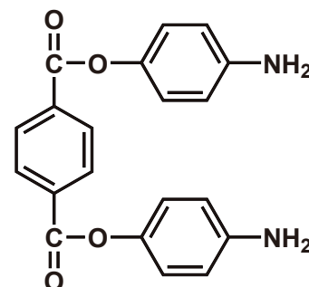
BPTP
