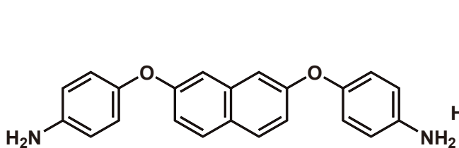
ET-2,7-Na
