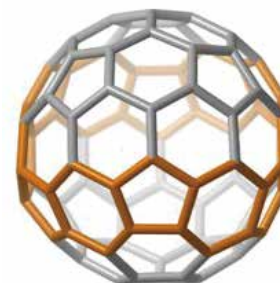
I_h - C_{80}
