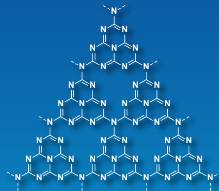
g-C 3 N 4
