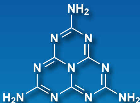
Melem
