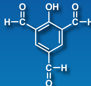
2-Hydroxy-1,3,5-benzenetricarbaldehyde
