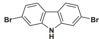
2,7-Dibromocarbazole
