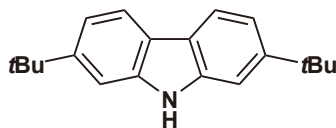
2,7-Di-tert-butyl-9H-carbazole
