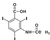
Acetrizic acid
