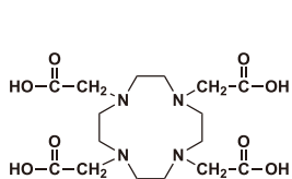
DOTA
