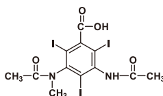
Metrizic acid
