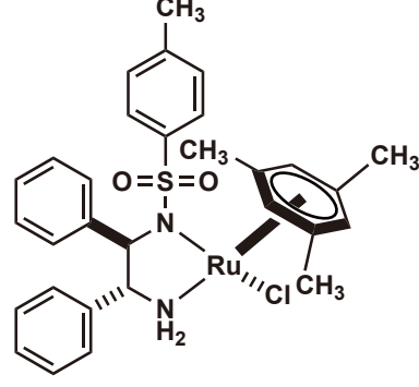
RuCl[(R,R)-Tsdpen](mesitylene)
