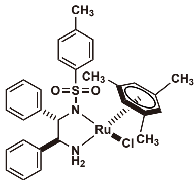
RuCl[(S,S)-Tsdpen](mesitylene)
