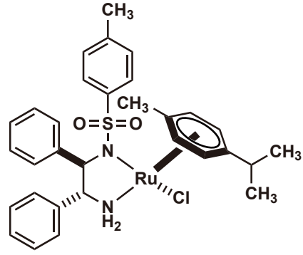
RuCl[(R,R)-Tsdpen](p-cymene)
