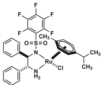
RuCl[(R,R)-Fsdpen](p-cymene)
