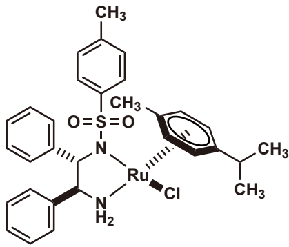
RuCl[(S,S)-Tsdpen](p-cymene)
