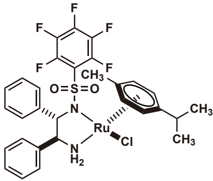
RuCl[(S,S)-Fsdpen](p-cymene)
