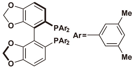
(R)-(+)-DM-SEGPHOS®
