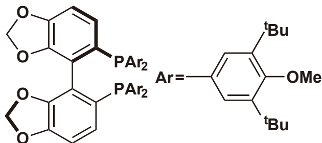
(R)-(-)-DTBM-SEGPHOS®
