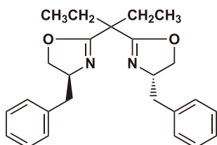
( S,S )-3,3-Bis(4-benzyl-2-oxazolin-2-yl)pentane
