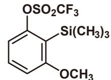
3-Methoxy- 2-(trimethylsilyl)phenyl Trifluoromethanesulfonate 1g 14,400円 / 5g 46,100円 [M1884]
