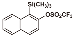
1-(Trimethylsilyl)-2-naphthyl Trifluoromethanesulfonate 1g 19,400円 / 5g 65,600円 [T2465]
