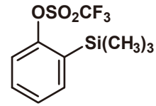
2-(Trimethylsilyl)phenyl Trifluoromethanesulfonate 1g 7,300円 / 5g 22,500円 / 25g 75,100円 [T2089]
