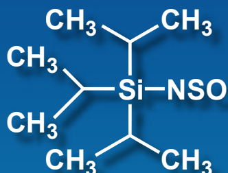
N-Sulfinyltriisopropylsilylamine (= TIPS-NSO)
